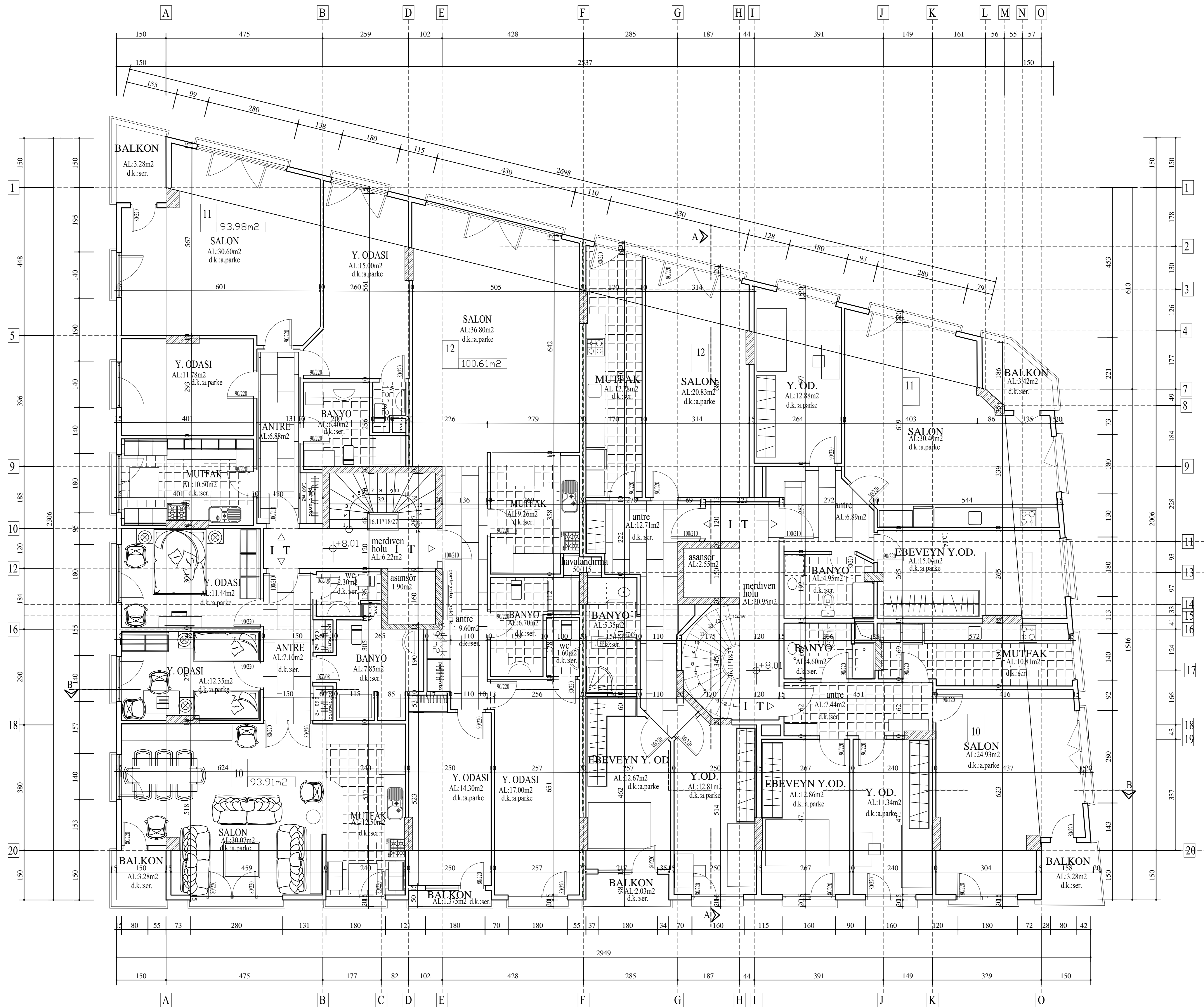
2.NORMAL KAT PLANI Ö=1/50
